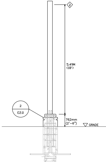
4 TYPICAL POLE DETAIL E-4 SCALE: N.T.S.
